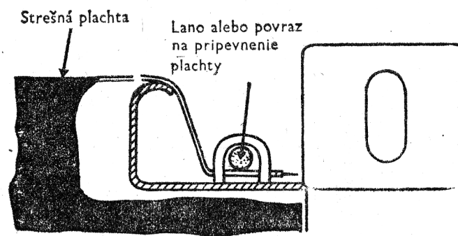
Vyobrazenie v reze
